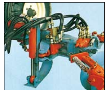
Slitta idraulica di regolazione profondità di lavoro Hydraulic skid to adjust the depth Hydraulischer Kufe zur Einstellung der Arbeitstiefe Glissière hydraulique de réglage profondeur de travail Guía hidráulica de regulación profundidad de trabajo
